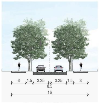
K-K道路横断面
