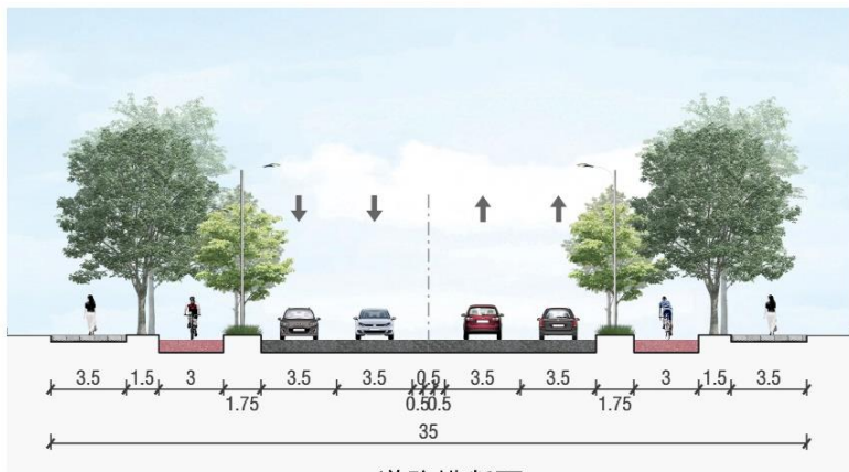
D-D道路横断面
