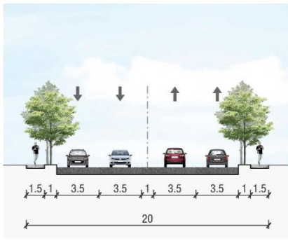
I-I道路横断面
